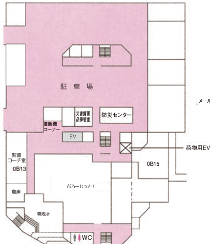
地階
